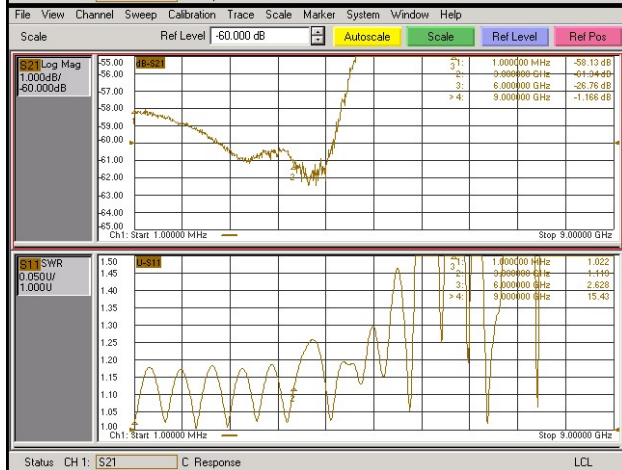
Графики для АЧХ - Log Mag, при отсчётом уровне равном -60 дБ, и для КСВ - SWR
