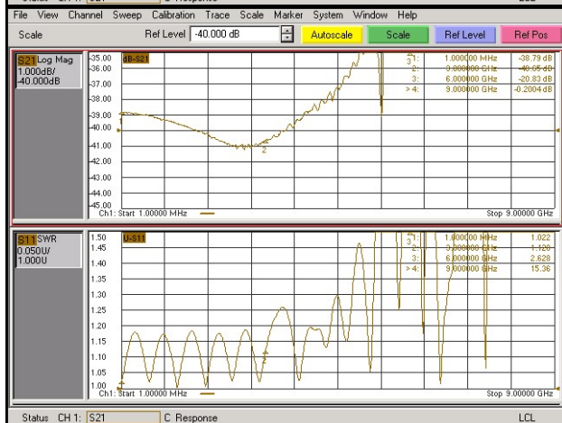
Графики для АЧХ - Log Mag, при отсчётом уровне равном -40 дБ, и для КСВ - SWR
