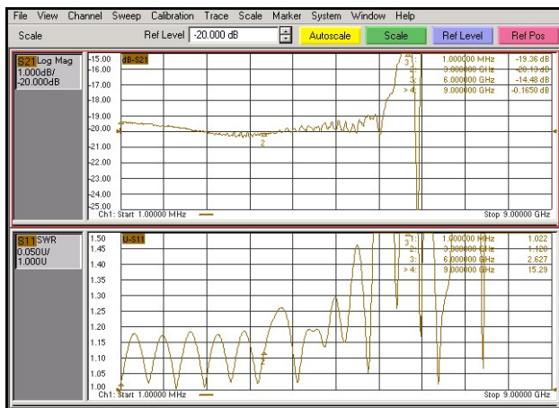
Графики для АЧХ - Log Mag, при отсчётом уровне равном -20 дБ, и для КСВ - SWR
