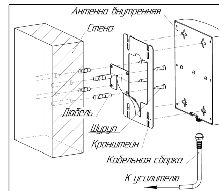
Схема 2 – Монтаж внутренней антенны
