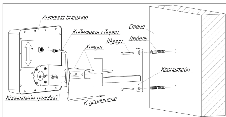
Схема 1 – Монтаж антенны на кронштейн КН-200
